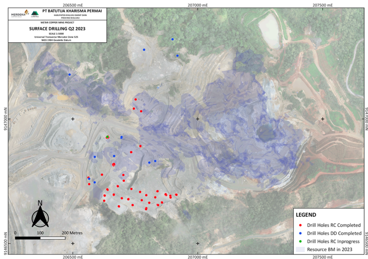
Gambar 4: Status lubang bor RC dan DD di Partolang - Triwulan 2 2023
