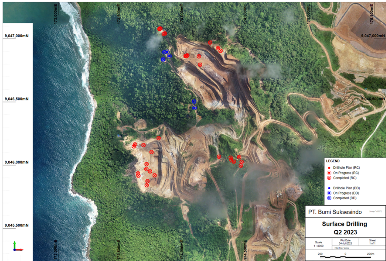
Gambar 3: Peta Pengeboran permukaan di Tujuh Bukit - Triwulan 2 2023
