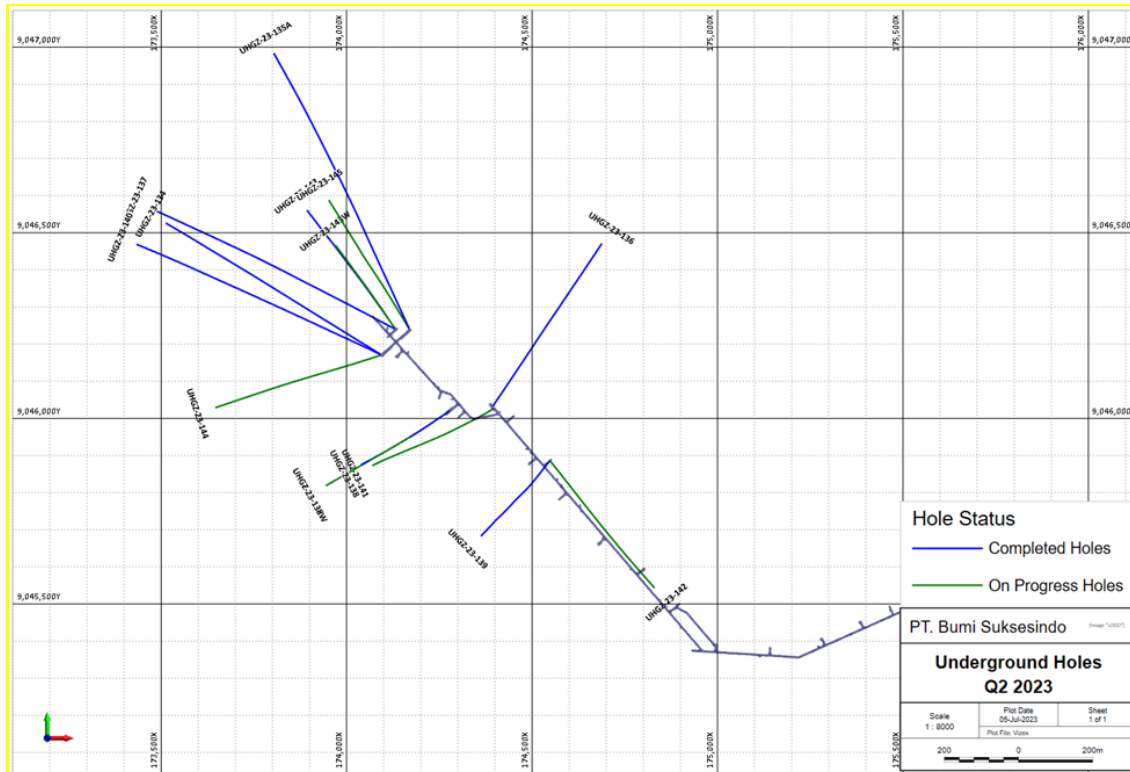
Gambar 2: Tuhuh Bukit – lubang bor bawah permukaan - Triwulan 2 2023
