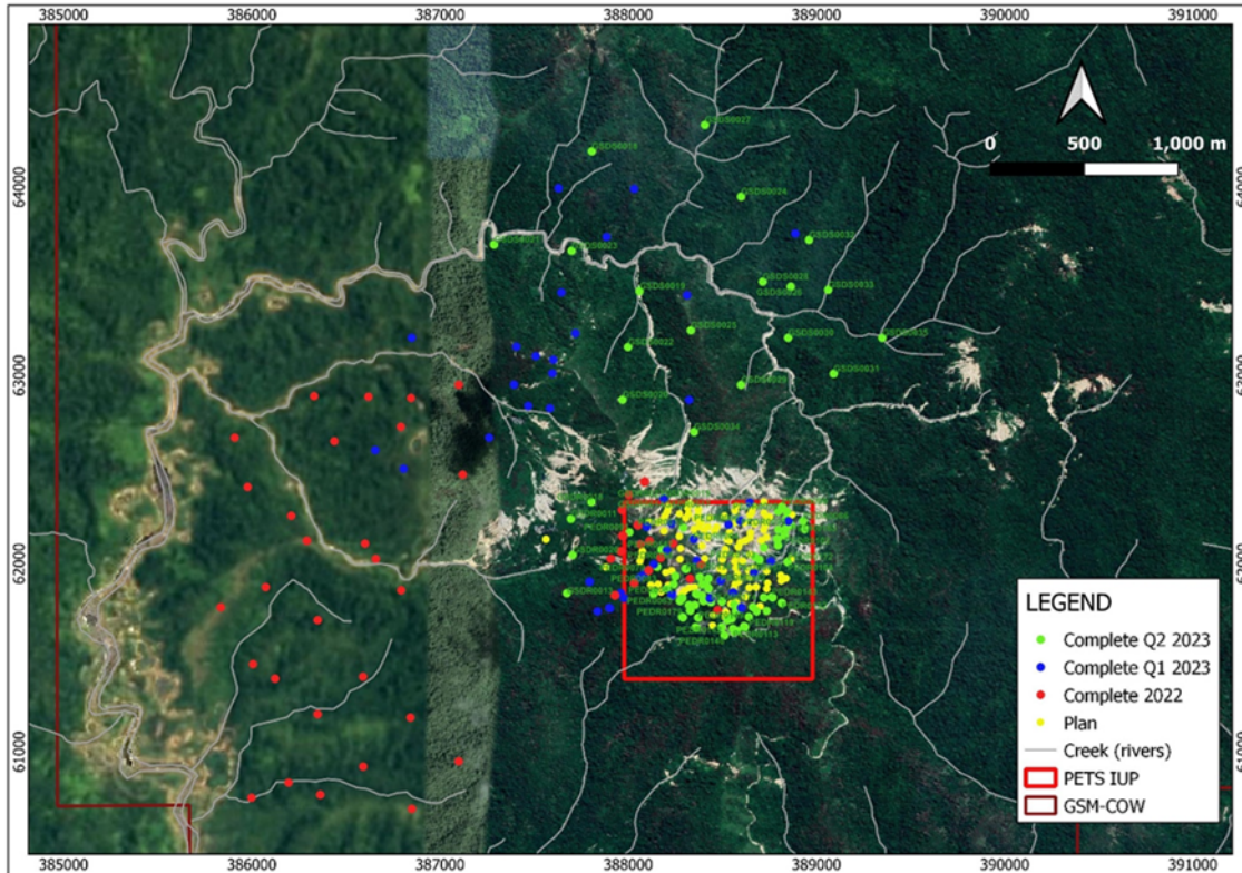
Gambar 5: Peta rencana lubang bor dan yang telah selesai diatas topografi – Triwulan 2 2023
