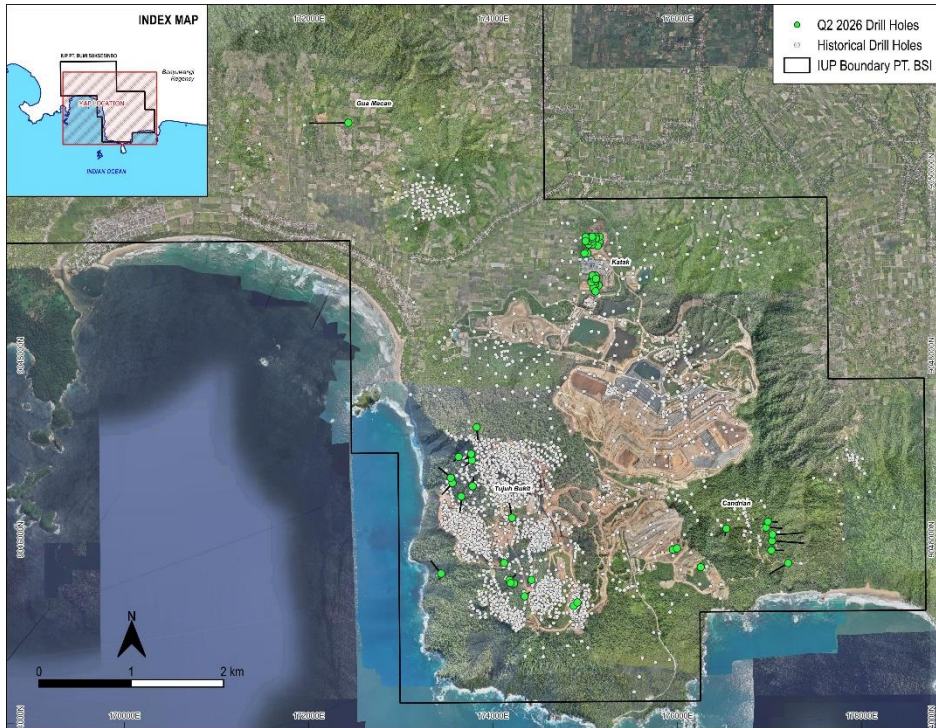
Gambar 2: Peta Lokasi Pengeboran Permukaan Tujuh Bukit pada Q2 2026 Figure 2: Tujuh Bukit Surface Drilling Locations in Q2 2026
